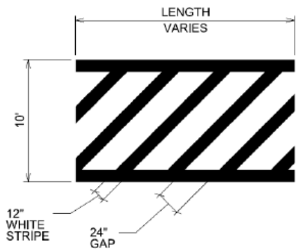
"DIAGONAL STYLE" CROSSWALK N.T.S.
