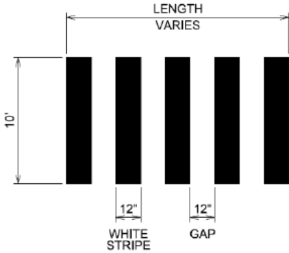
"CONTINENTAL STYLE" CROSSWALK N.T.S.
